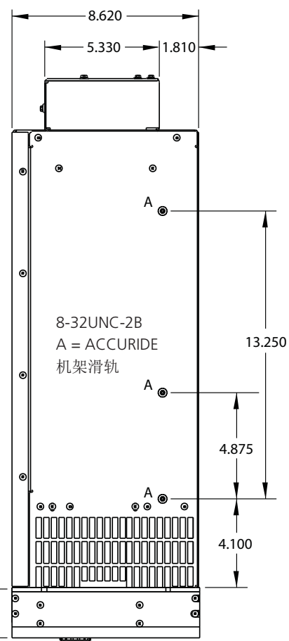
侧视图
