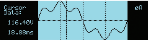
电压采集波形（CSW显示屏）。
