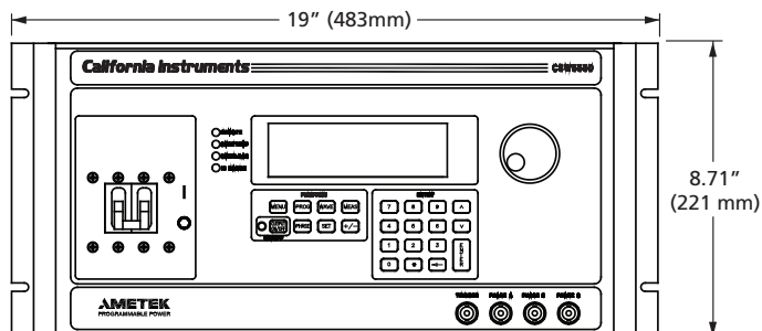
正视图
