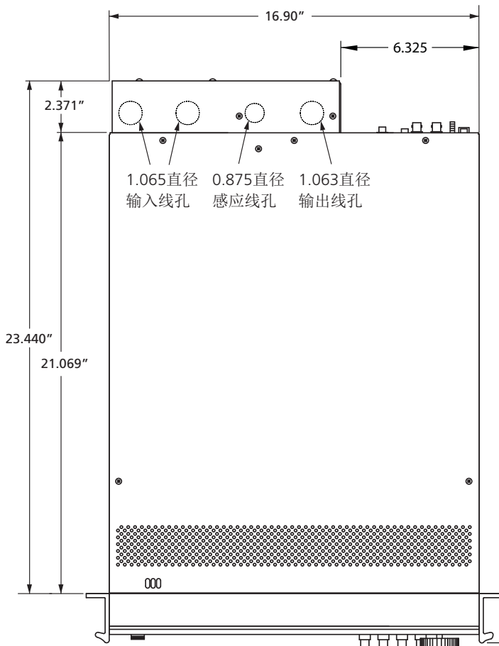
俯视图
