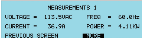
单相测量数据（BPS显示屏）。
