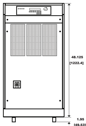
正视图
