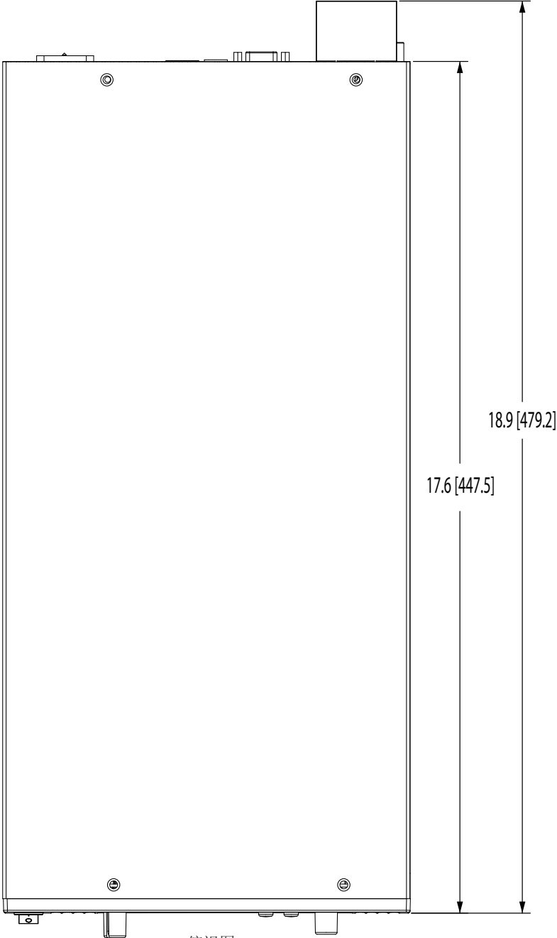
俯视图
