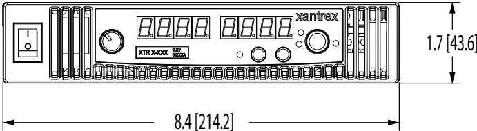
正视图
