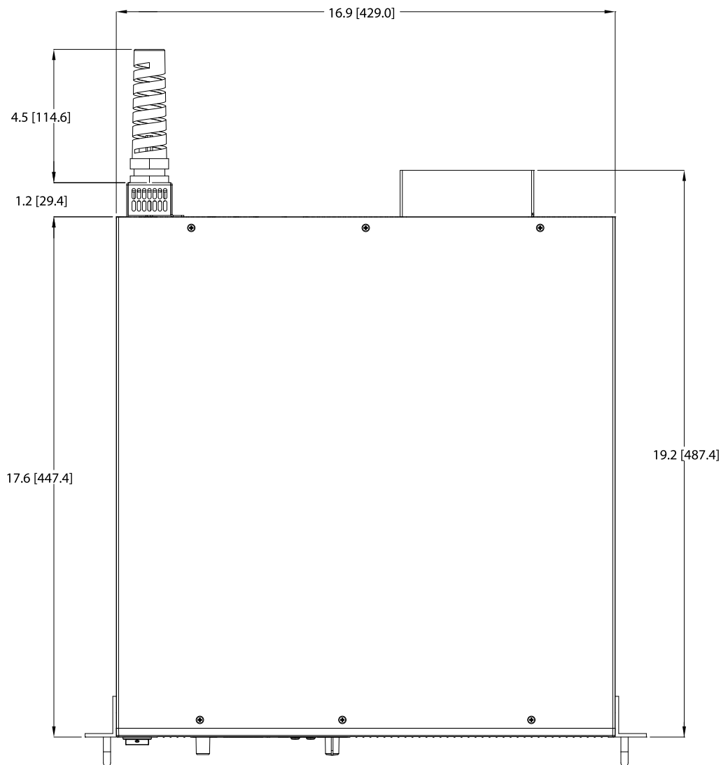
俯视图
